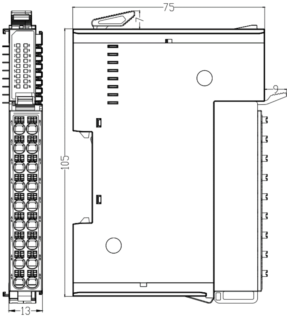
正视
